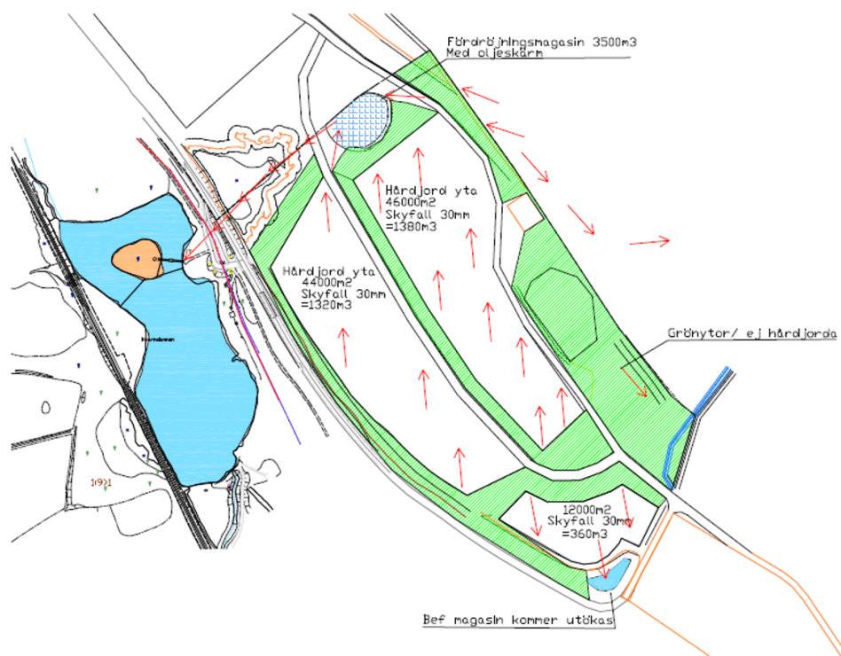
Figur 8: Illustration av föreslagen dagvattenlösning
